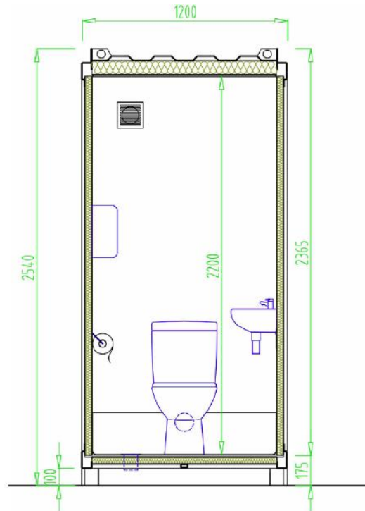
Innenansicht vorne
